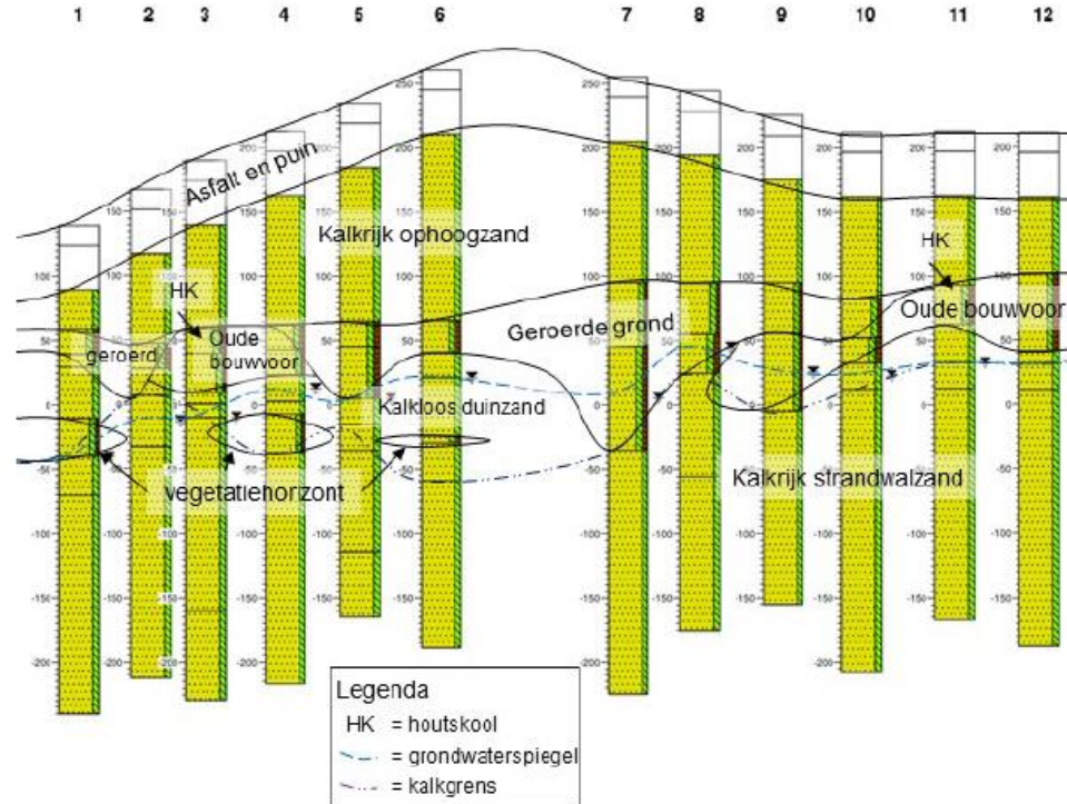
Figuur 2: schematische doorsnede van de bodem op basis van de boringen.
